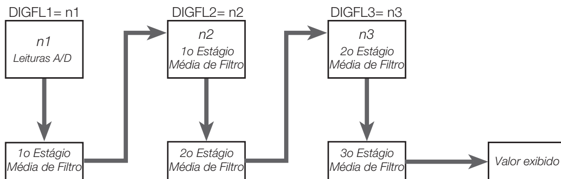
Figura 7-3. Diagrama de fluxo para CW-90/90X filtros digitais
