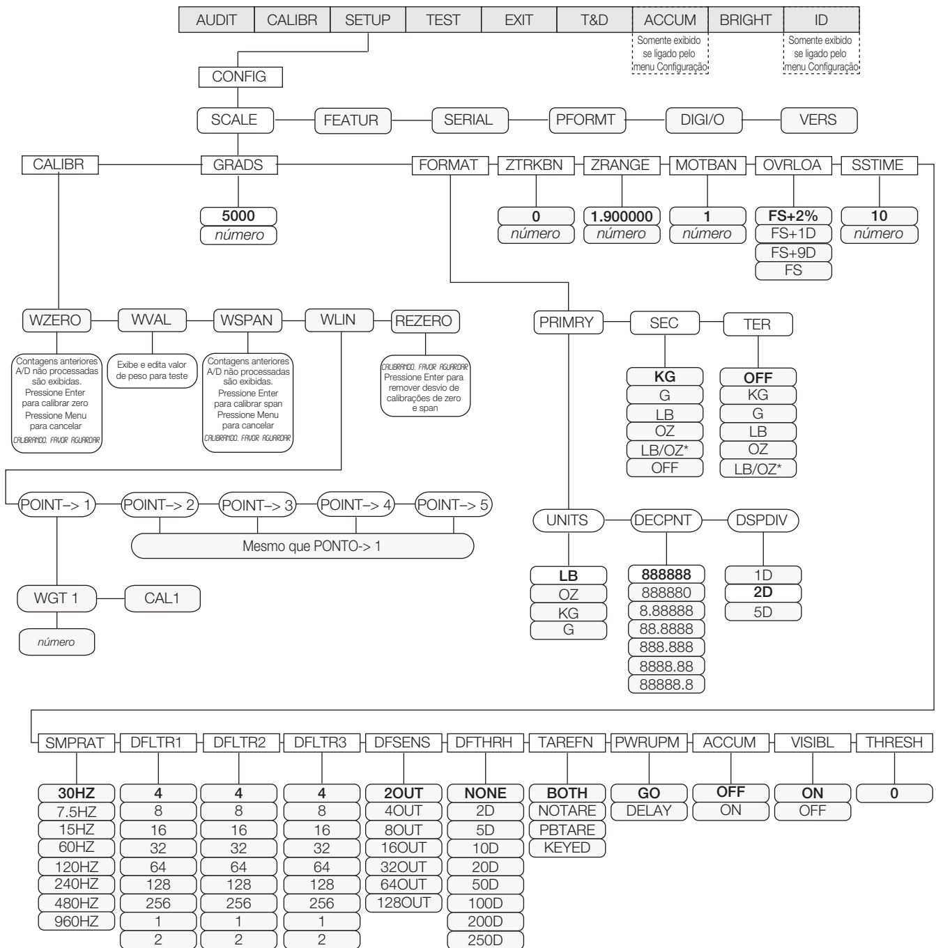
Figura 3-5. Menu Configuração: Submenu Balança
