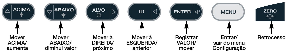
Figura 3-2. Funções da tecla do painel frontal no modo menu
